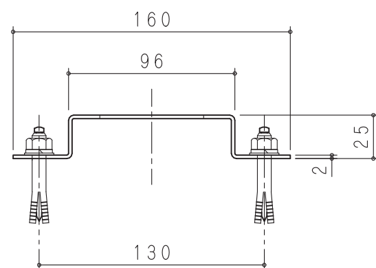
A部拡大図 (S=1/3)
