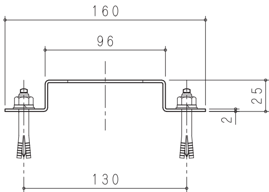
A部拡大図 (S=1/3)
